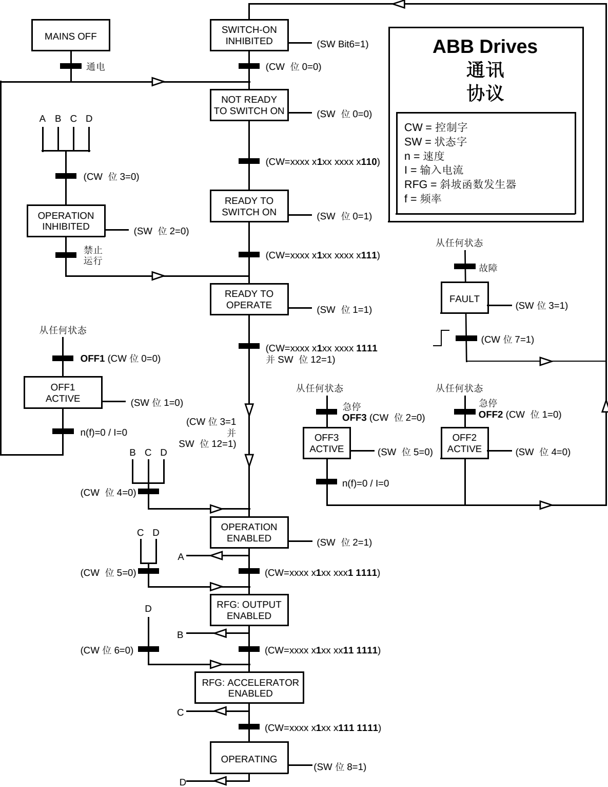
图1 ABB Drives 通讯协议的状态机器
